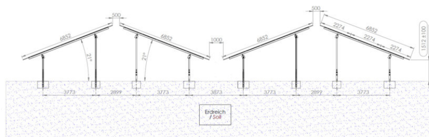
Prinzipische Skizze 1 Modultische; Quelle: WIRCON GmbH, Konrad-Zuse-Ring 30, 68163 Mannheim
