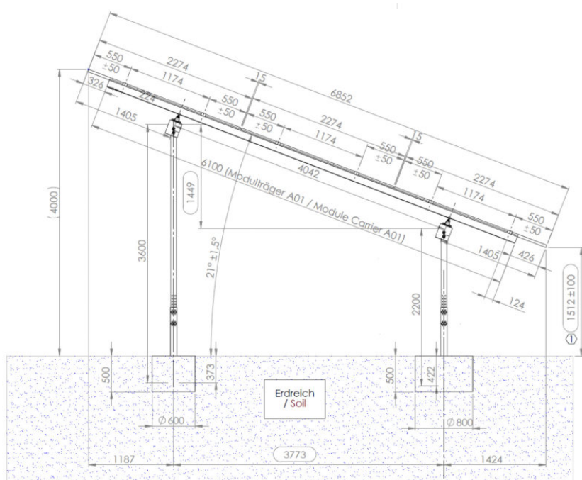
Prinzipische Skizze 2 Modultisch; Quelle: WIRCON GmbH, Konrad-Zuse-Ring 30, 68163 Mannheim
