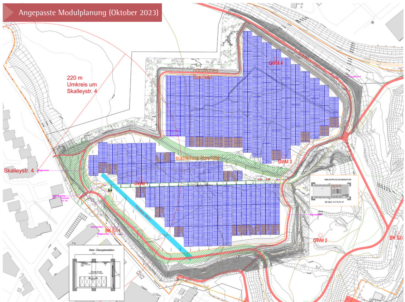
Vorhaben- und Erschließungsplan mit Detailzeichnungen; Quelle: WIRCON GmbH, Konrad-Zuse-Ring 30, 68163 Mannheim; ohne Maßstab
