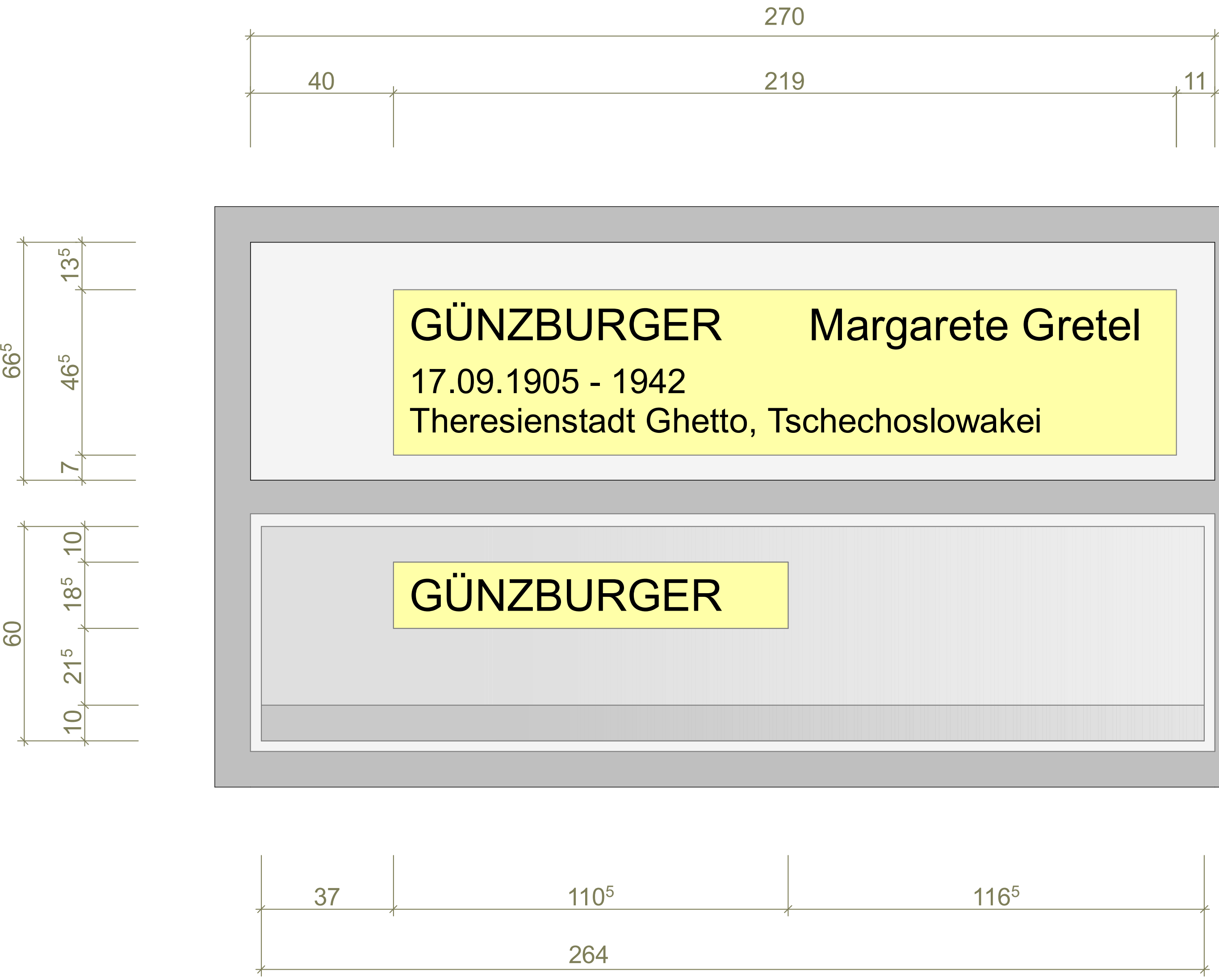
Detail Briefkasten M 1:1 / Maße in mm
